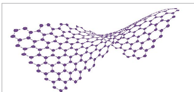
Схематическое изображение графена
